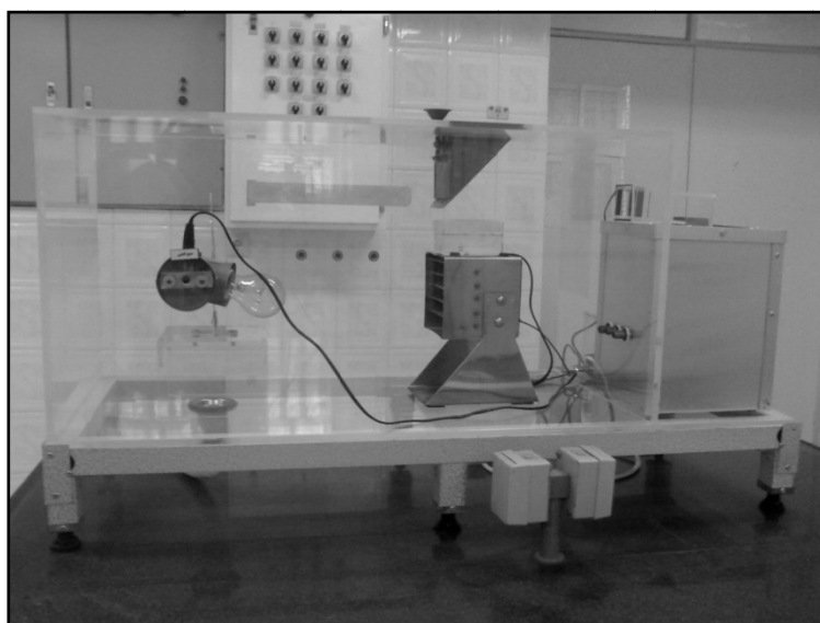
شکل ۱: محفظه شبیه سازی آلاینده‌های هواپرد
